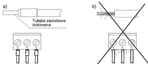
Zabezpieczanie końców przewodów: a) prawidłowe, b) nieprawidłowe.
